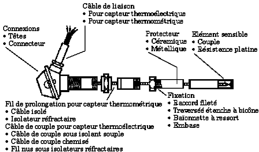
Figure 1 : Structure d'un capteur électrique (source : http://perso.club-internet.fr/gatt/ ).
