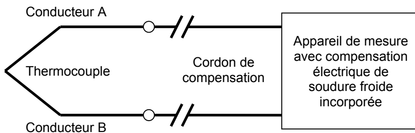
Figure 2 : exemple de montage d'un thermocouple
